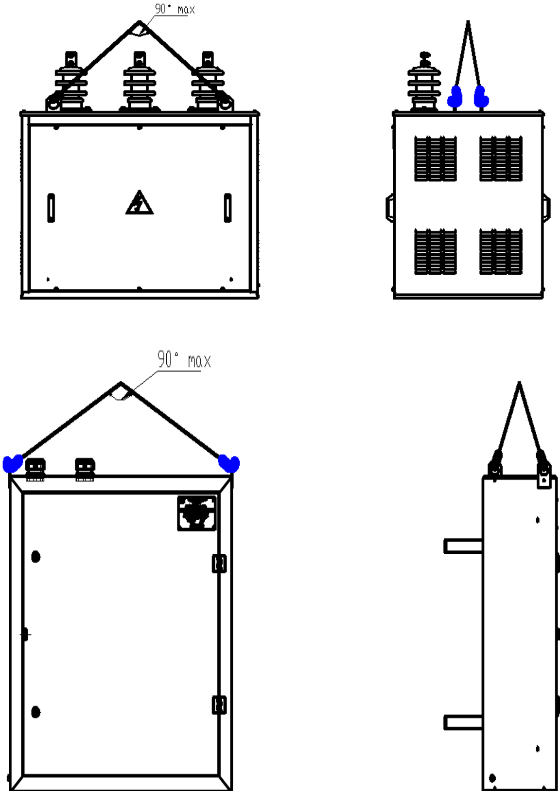
Схема строповки РУНН и модуля тр-ра
