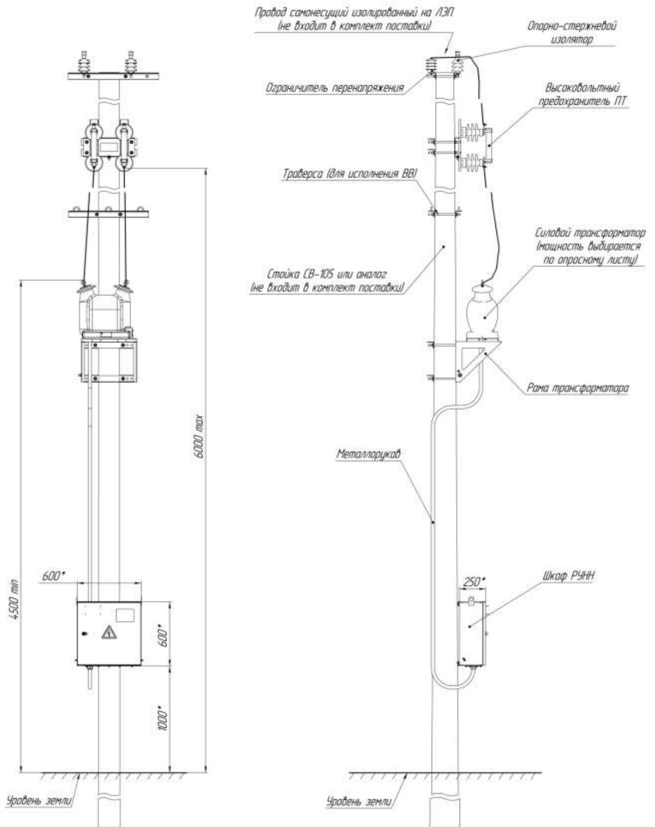
Рис. Б2 Внешний вид однофазной КТПС
