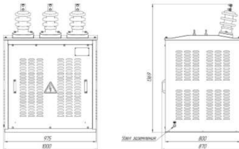
Рис. Г1 Внешний вид и габариты модуля трансформатора ТЛС, мощностью 25 кВ·А; 40 кВ·А и 63 кВ·А
