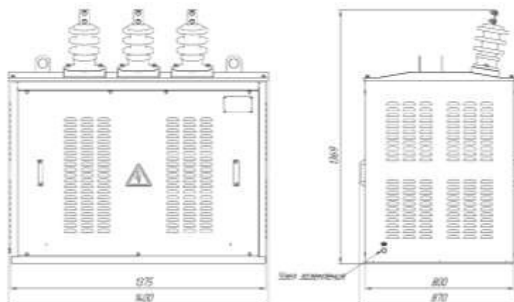
Рис. Г2 Внешний вид и габариты модуля трансформатора ТЛС, мощностью 100 кВ·А
