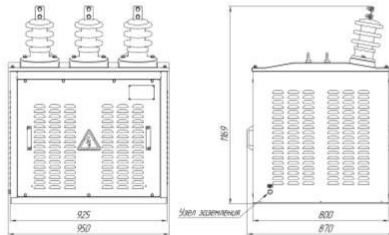
Рис. Г1 Внешний вид и габариты модуля трансформатора ТЛС, мощностью 25 кВ·А; 40 кВ·А и 63 кВ·А
