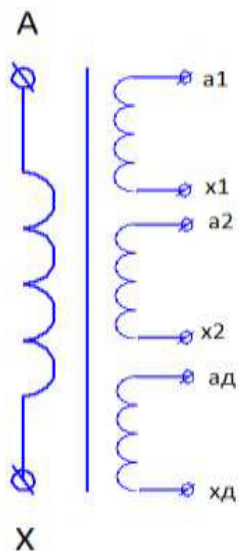
Рисунок 1 - Схема включения
