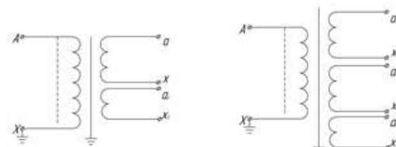
Рисунок А.7 Принципиальная электрическая схема трансформатора ЗНОЛ-35(27) III
