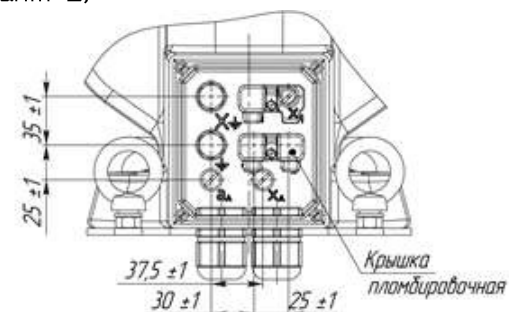
Рисунок А.6 Клеммник для трансформаторов ЗНОЛ-35 (остальное см. рисунок А.5, крышка условно не показана)
