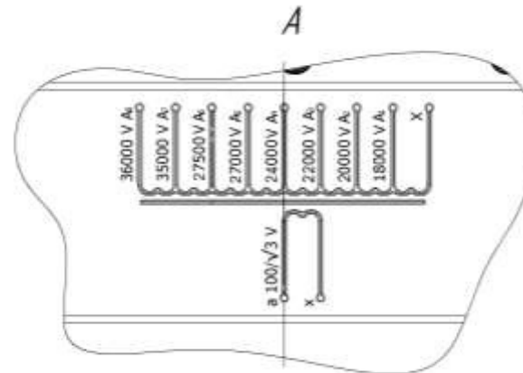
Рисунок А.10 Габаритные, установочные, присоединительные размеры и масса трансформаторов Н/Л-35-4 (остальное — см. рисунок А.6)
