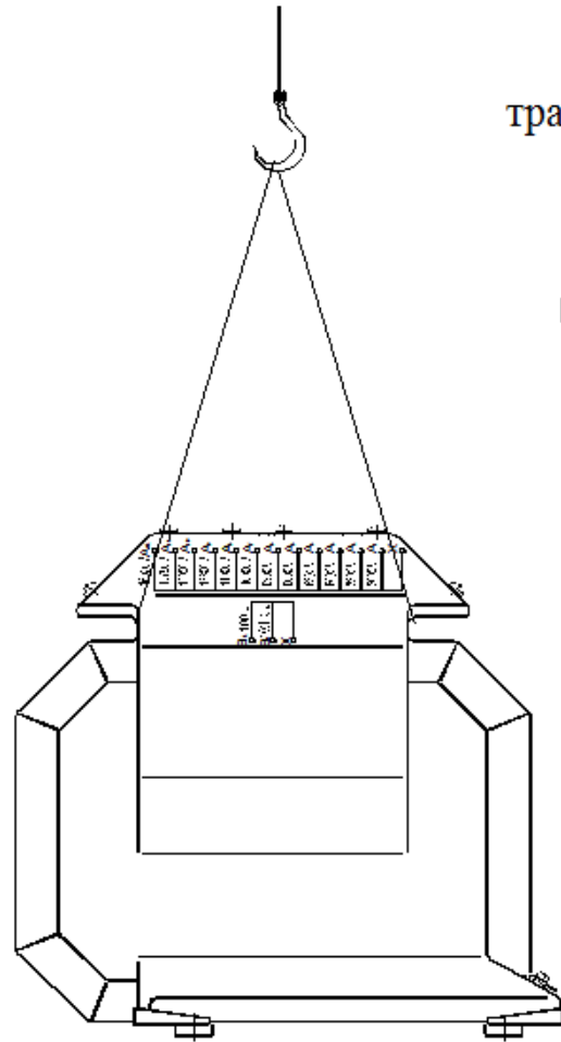
Рисунок Б.1 Способ строповки №1
