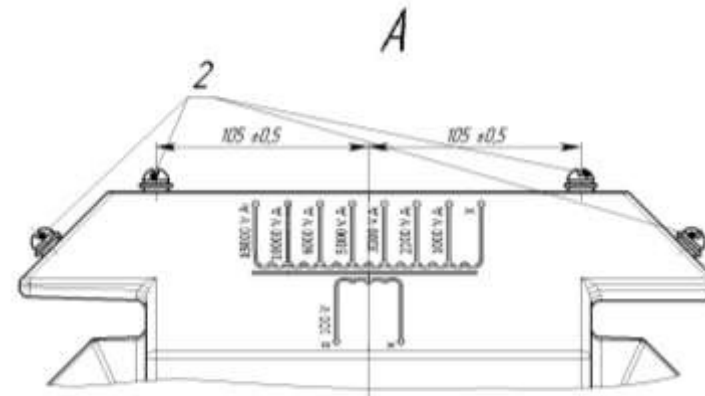
Рисунок А.4 Габаритные, установочные, соединительные размеры и масса трансформаторов Н/Л-15-3 (остальное – см. рисунок А.1)
