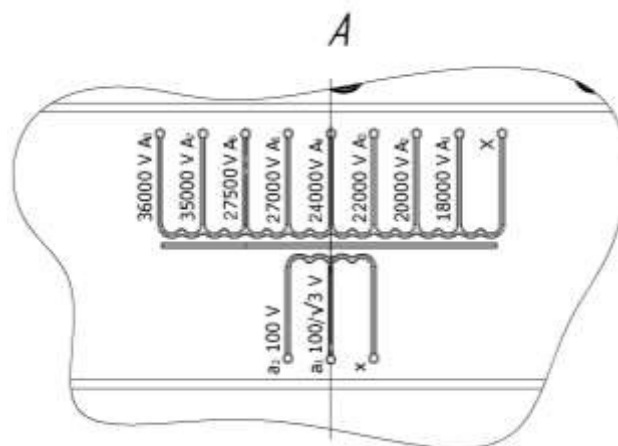
Рисунок А.7 Габаритные, установочные, соединительные размеры и масса трансформаторов Н/Л-35-1 (остальное – см. рисунок А.6)
