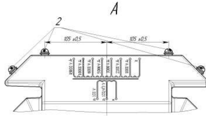
Рисунок А.4 Габаритные, установочные, соединительные размеры и масса трансформаторов Н/Л-15-3 (остальное – см. рисунок А.1)
