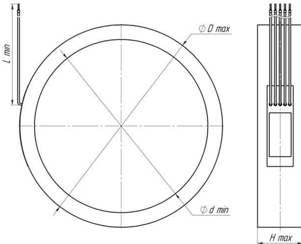
Рисунок Б.1 – ТВ-330-I; ТВ-500-I; ТВ-750-I; ТВ-750-II
