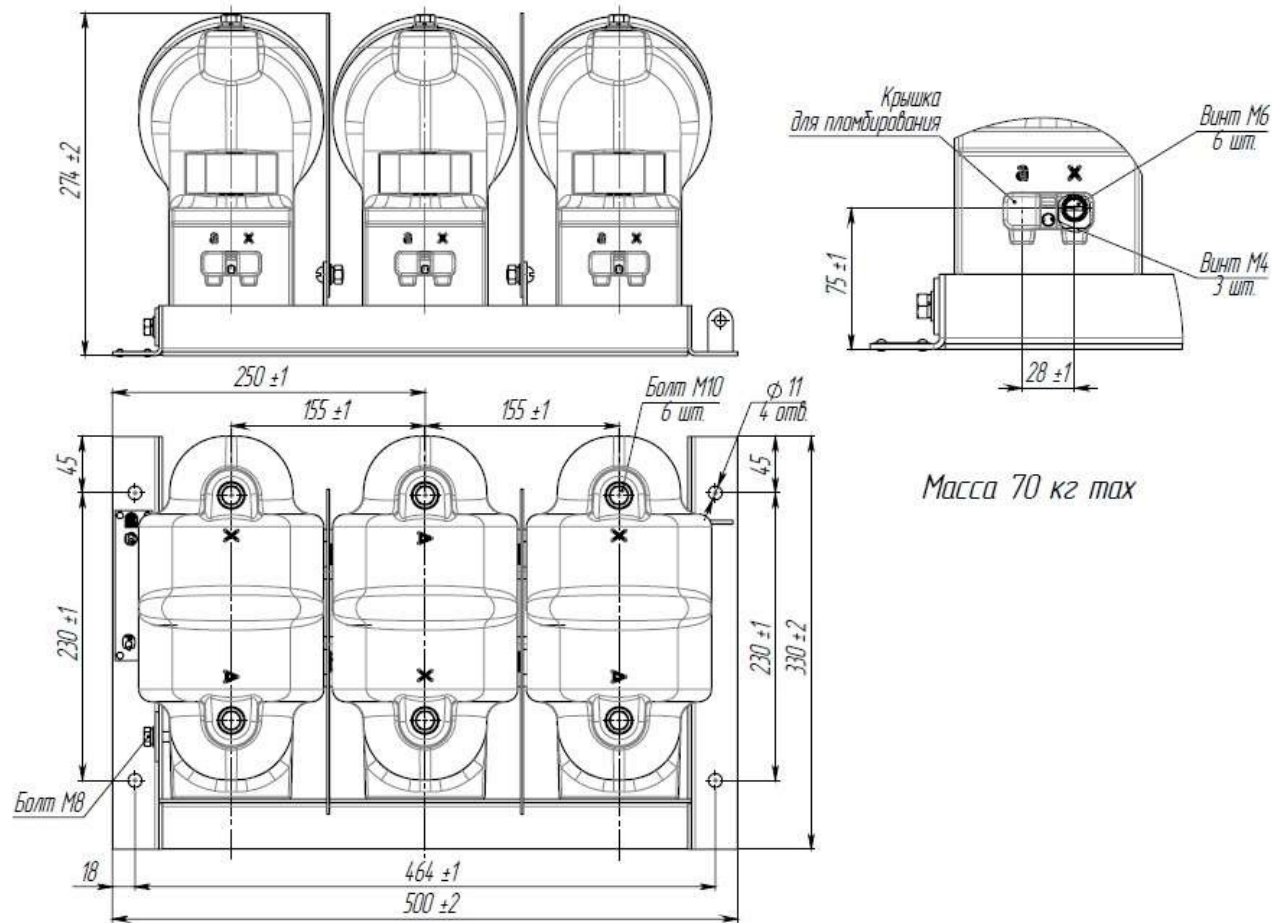
Рисунок А.1 Общий вид трехфазной группы трансформаторов напряжения НОЛ.08-6(10)М
