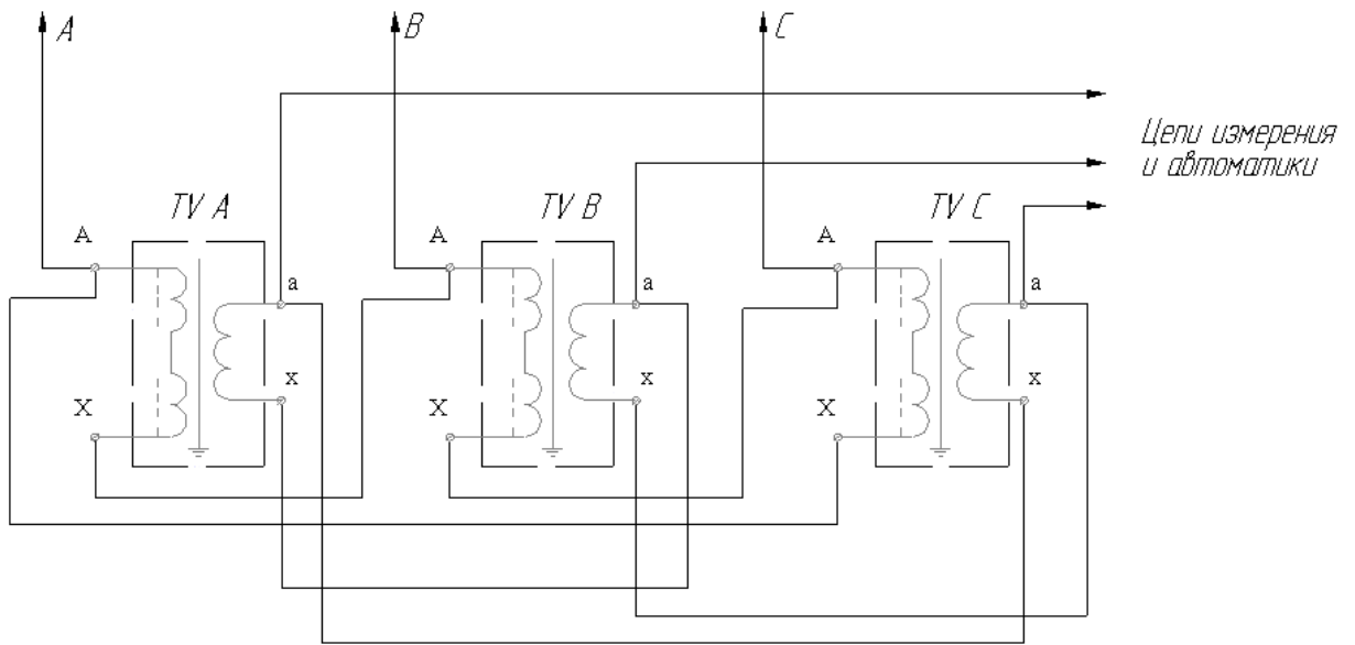
Рисунок А.2 Принципиальная электрическая схема трехфазной группы
