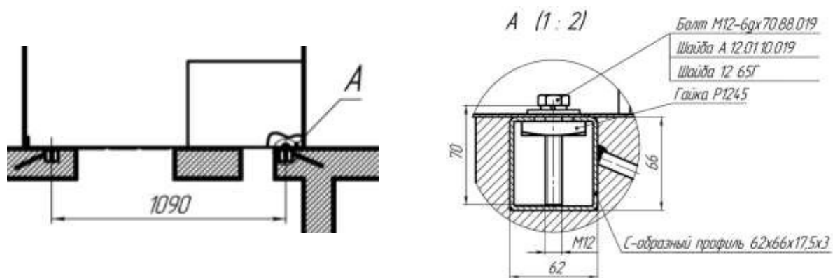
Рисунок 11 – Способ крепления шкафа к закладным основания
