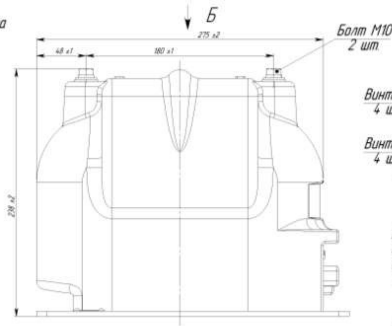
Рисунок Б.2 Расположение низковольтных вводов НОЛ.08.3-6(10)М
