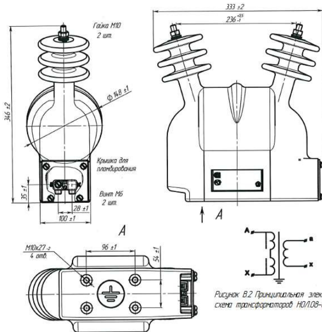
Рисунок В.1 Общий вид трансформаторов НОЛ.08-6(10)М IV
