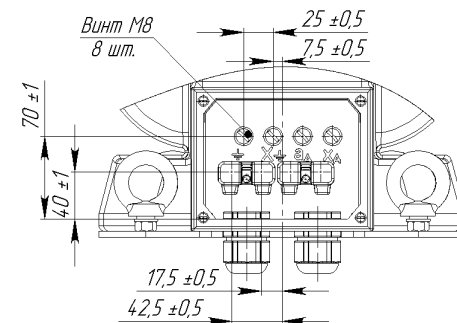
Рисунок А.2 Клеммник для трансформаторов ЗНОЛ-35 III (остальное см. рисунок А.1, крышка условно не показана)
